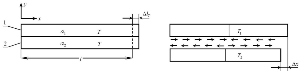
Рисунок 9 – Формування дотичних напружень у двошаровому брусі
