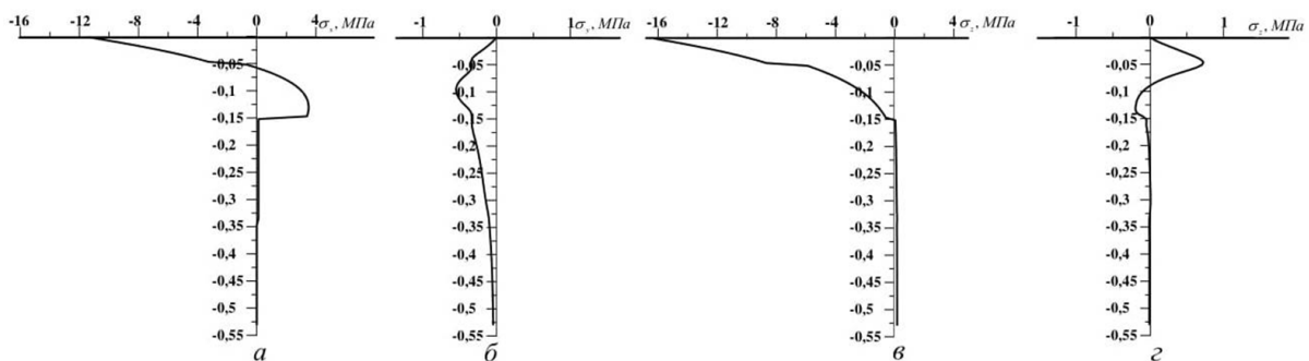
Рисунок 11 – Графіки функцій \sigma_x(y) (а), \sigma_y(y) (б), \sigma_z(y) (в), \tau_{xy} (г) при t = 6 \text{ год} і T = -25^{\circ}\text{C}
