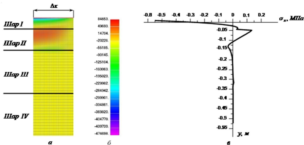
Рисунок 5 – Графіки функцій \sigma_x(y) в смужці \Delta x центральної зони перерізу z = 0 дорожнього одягу (а, б) та вздовж осі Oy (в) в момент t = 3200
