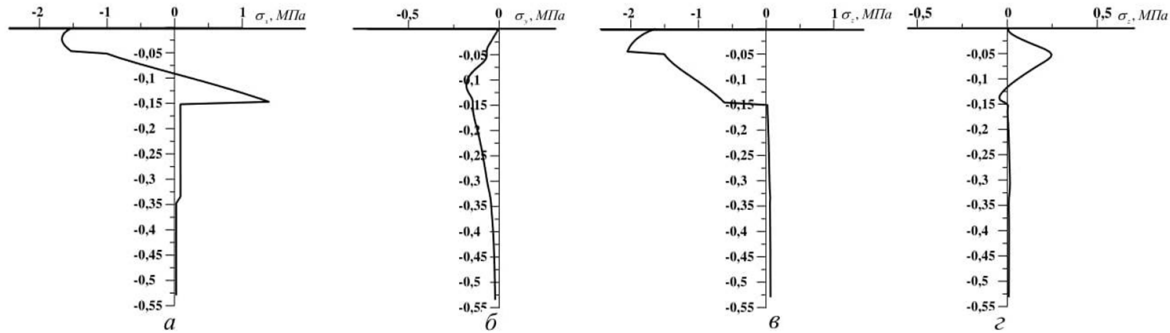
Рисунок 10 – Графіки функцій \sigma_x(y) (а), \sigma_y(y) (б), \sigma_z(y) (в), \tau_{xy} (г) при t = 6 \text{ год} і T = 25^{\circ}\text{C}
