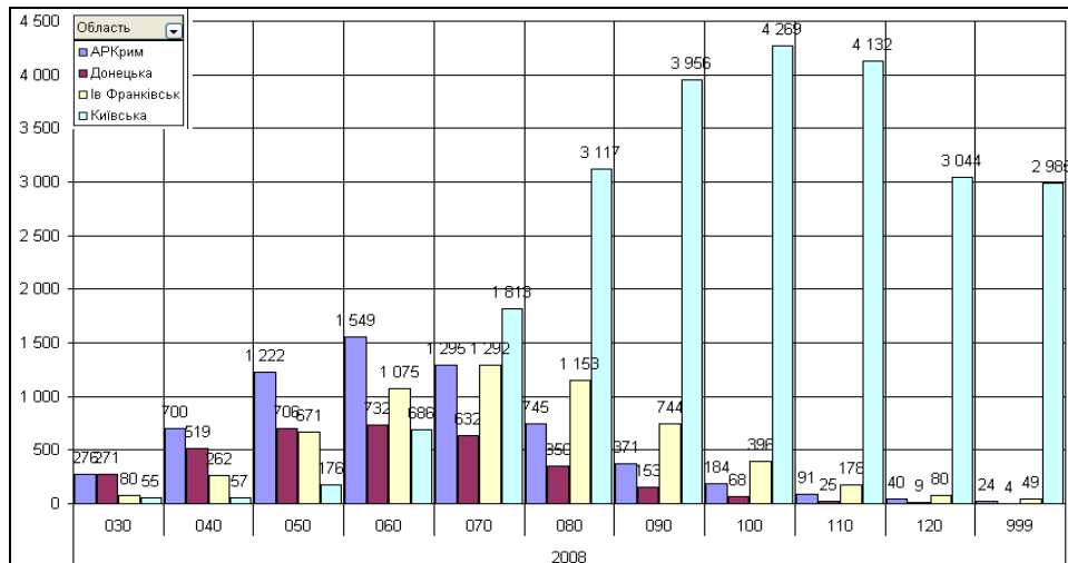
Рисунок 2.3 – Середні швидкості руху транспортних засобів в різних регіонах України за 2008 рік
