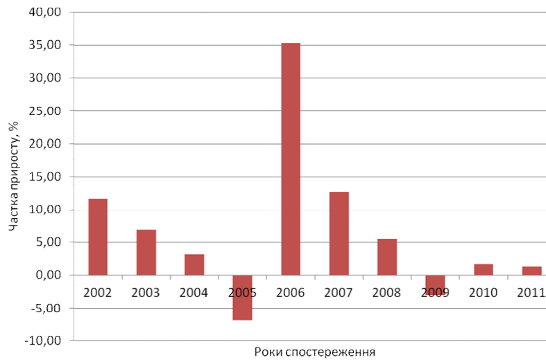
Рисунок 2.2 – Зміна середнього приросту інтенсивності руху на автомобільних дорогах державного значення
