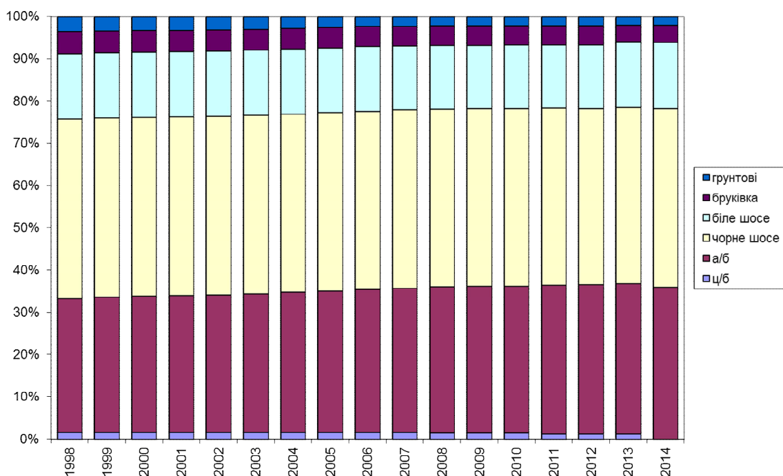
Рисунок 1.2 – Мережа автомобільних доріг України (розподіл за типами покриття)
