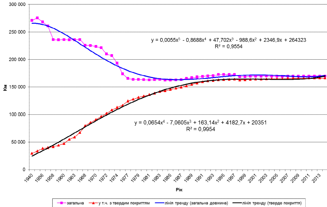
Рисунок 1.1 – Динаміка розвитку мережі автомобільних доріг України
